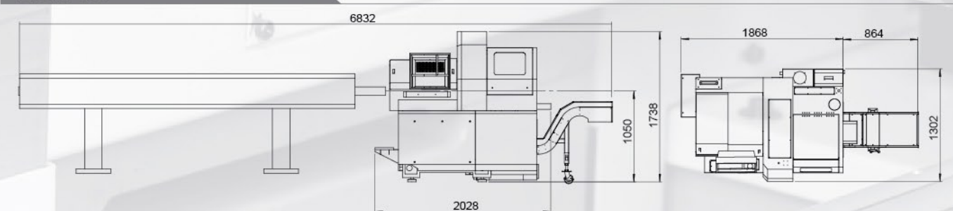
安装尺寸图 Installation Size (mm)
